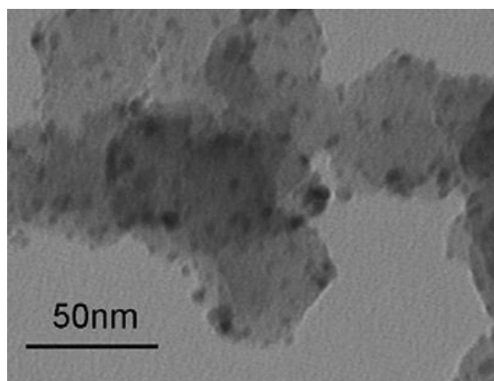
(4) 钯-钨催化剂，适于酸性电解液环境阴极氧气还原催化剂、碱性电解液环境阴极氧气还原催化剂、碱性电解环境乙醇氧化催化剂
