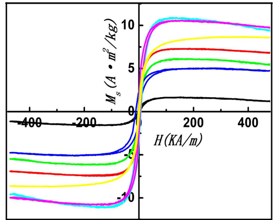
图 2 纤维的磁滞
