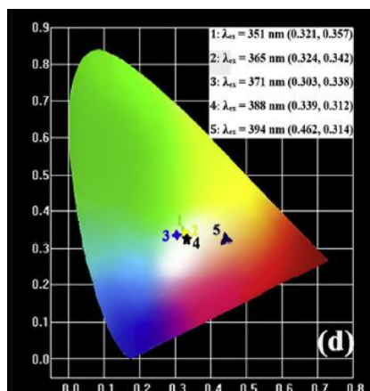
图 1 荧光粉 \text{NaCa}_{3.95}(\text{B}_3\text{O}_3)_3:0.02\text{Dy}^{3+}, 0.01\text{Tb}^{3+}, 0.02\text{Eu}^{3+} 在不同激发波长下的色坐标
