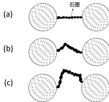
图 3 双芯之间石墨连接横断面示意图
