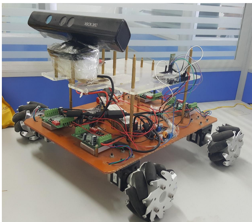
原型机图
